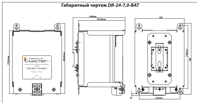
Габаритный чертёж DR-24-7,0-BAT
